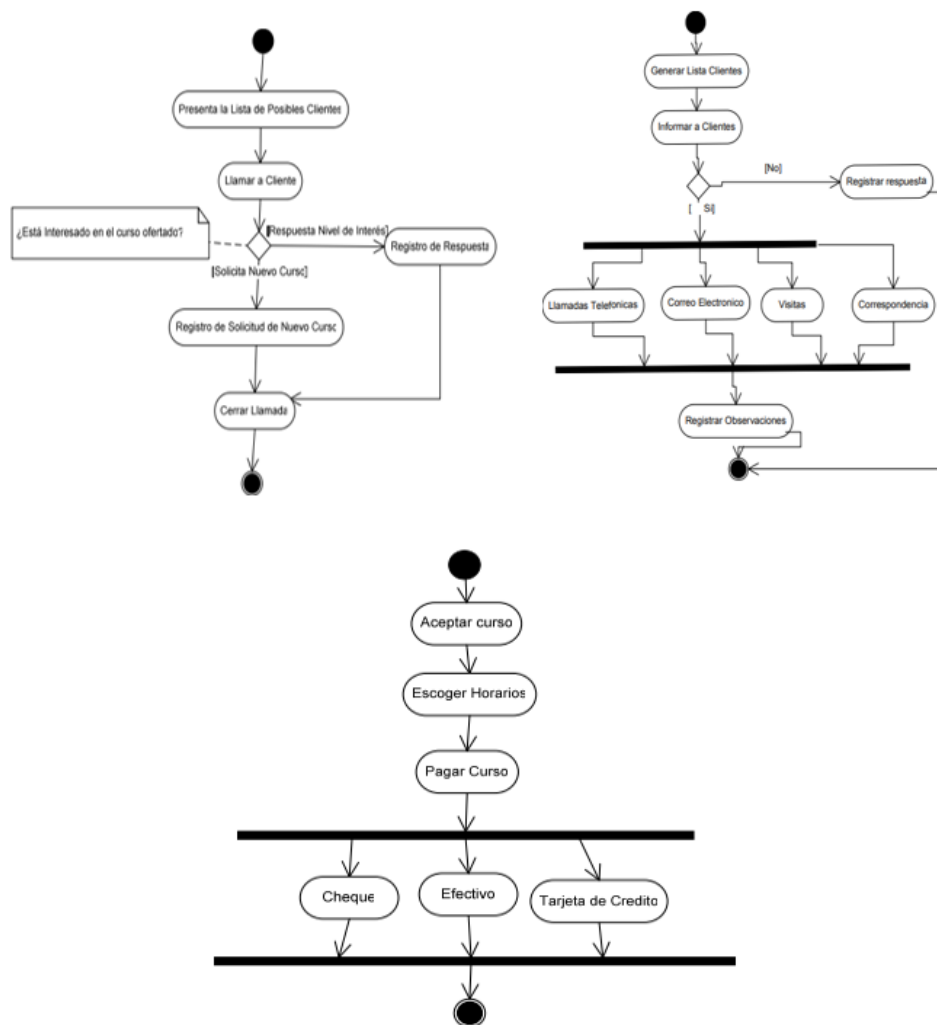
Figura 4. Diagrama de actividad del módulo CRM
