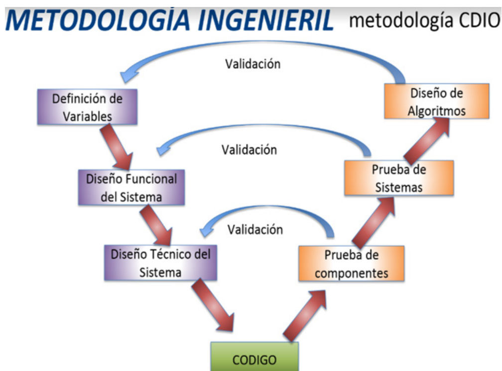
Figura 1. Metodología de desarrollo del sistema CRM. Elaboración propia.
